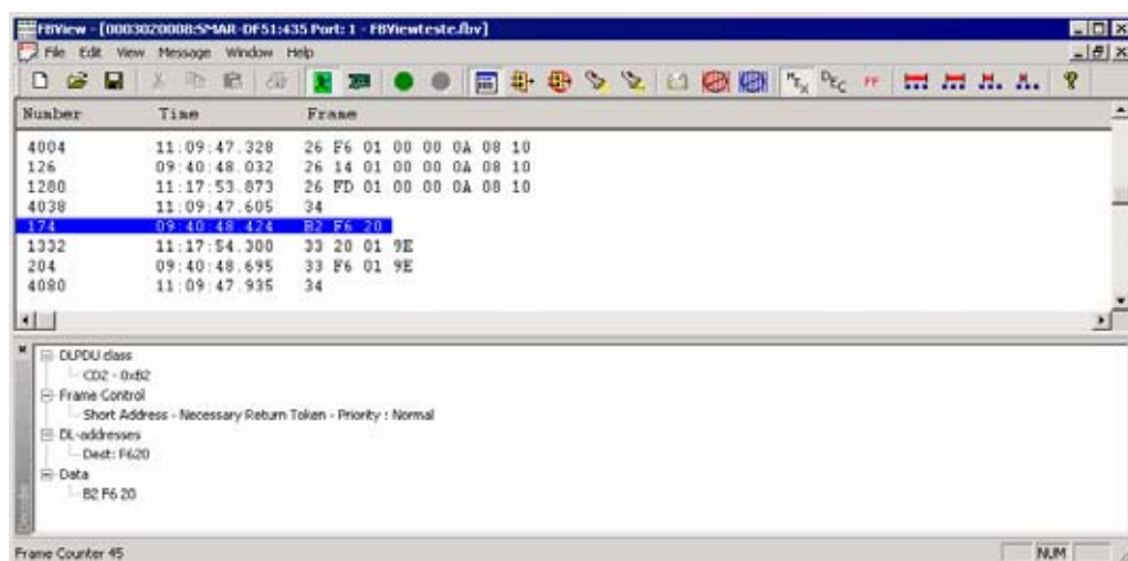
Figura 2.10. Mensagem Compel Data 2
