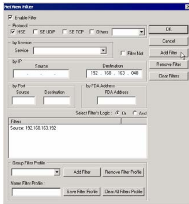
Figura 4.5. Criando um Filtro de Endereço de IP
