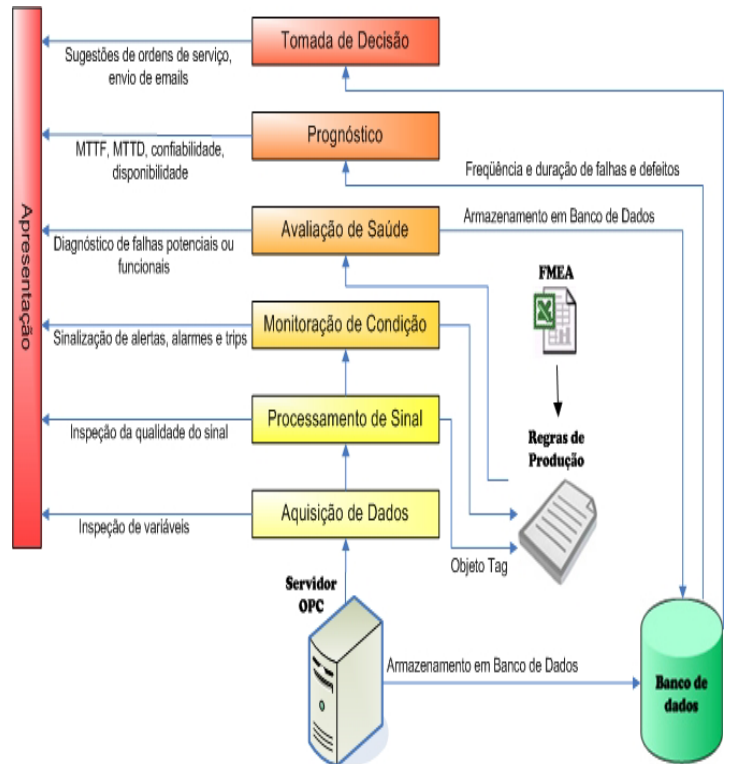
Figura 3. Fluxo de informações entre as camadas do sistema de manutenção preditiva.
