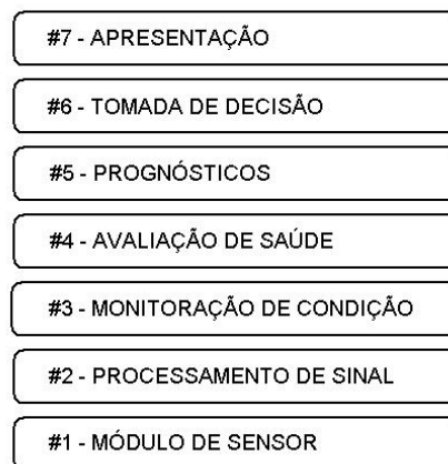
Figura1. Arquitetura OSA-CBM e suas 7 camadas.
