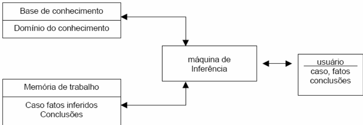
Figura 8.3: Sistema Especialista de 1º Geração
