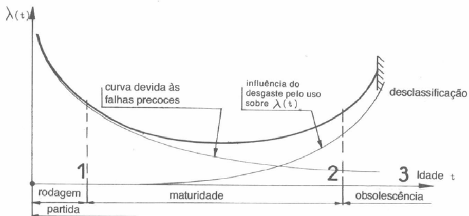
Figura 2.12 - Curva da Banheira – Equipamentos Mecânicos - Fonte: Monchy (1989, p. 81 )
