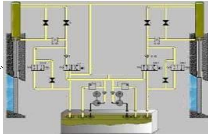
Assy: COMPORTA TOMADA D'ÁGU/ PN: FR: 1,43E-5 Qty: 1
