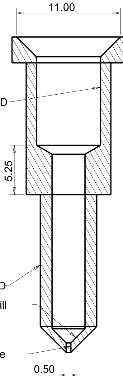
SECTION A-A
